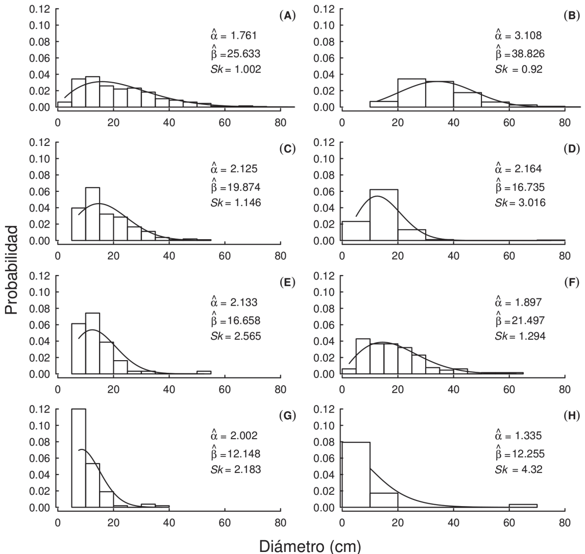
Fig. 2: Distribución diamétrica del bosque total (i.e., todas las especies) y por especies. La curva representa el ajuste de la función de Weibull \alpha = parámetro de escala, \beta = parámetro de forma y S_k = coeficiente de asimetría. Todos los ajustes fueron altamente significativos ( P < 0.0001 ). A) todas las especies, B) N. dombeyi , C) E. cordifolia , D) G. avellana , E) L. sempervirens , F) L. philippiana , G) A. punctatum , y H) P. saligna .
