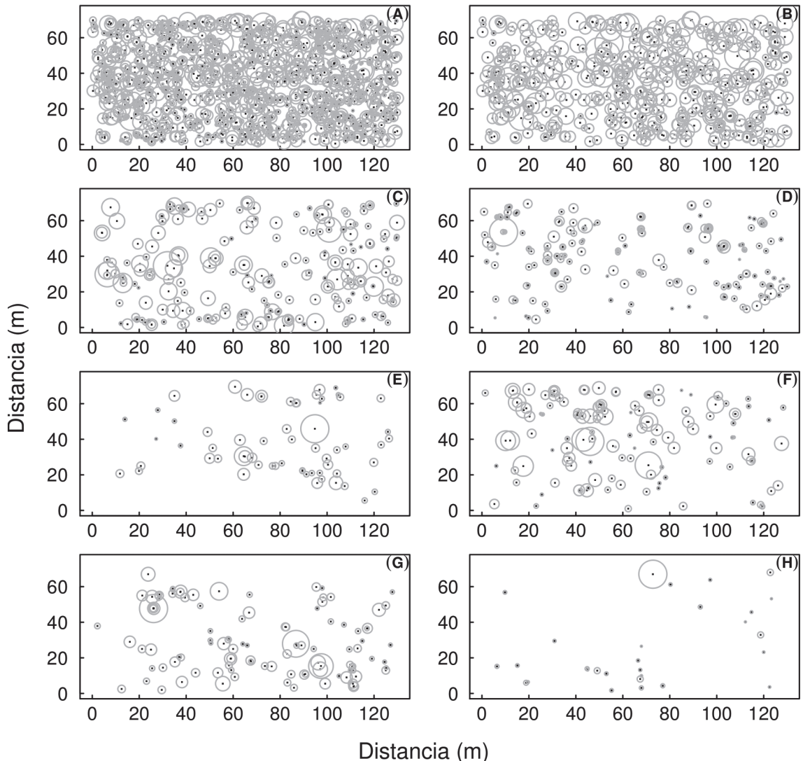
Fig. 1: Mapa de localización espacial de árboles en una parcela permanente de 70 x 130 m en el bosque de Llancahue, Chile. Figuras muestran los datos para A) todas las especies, B) N. dombeyi , C) E. cordifolia , D) G. avellana , E) L. sempervirens , F) L. philippiana , G) A. punctatum , and H) P. saligna . Círculos son proporcionales al d \times 100 en todos los árboles muestreados.
