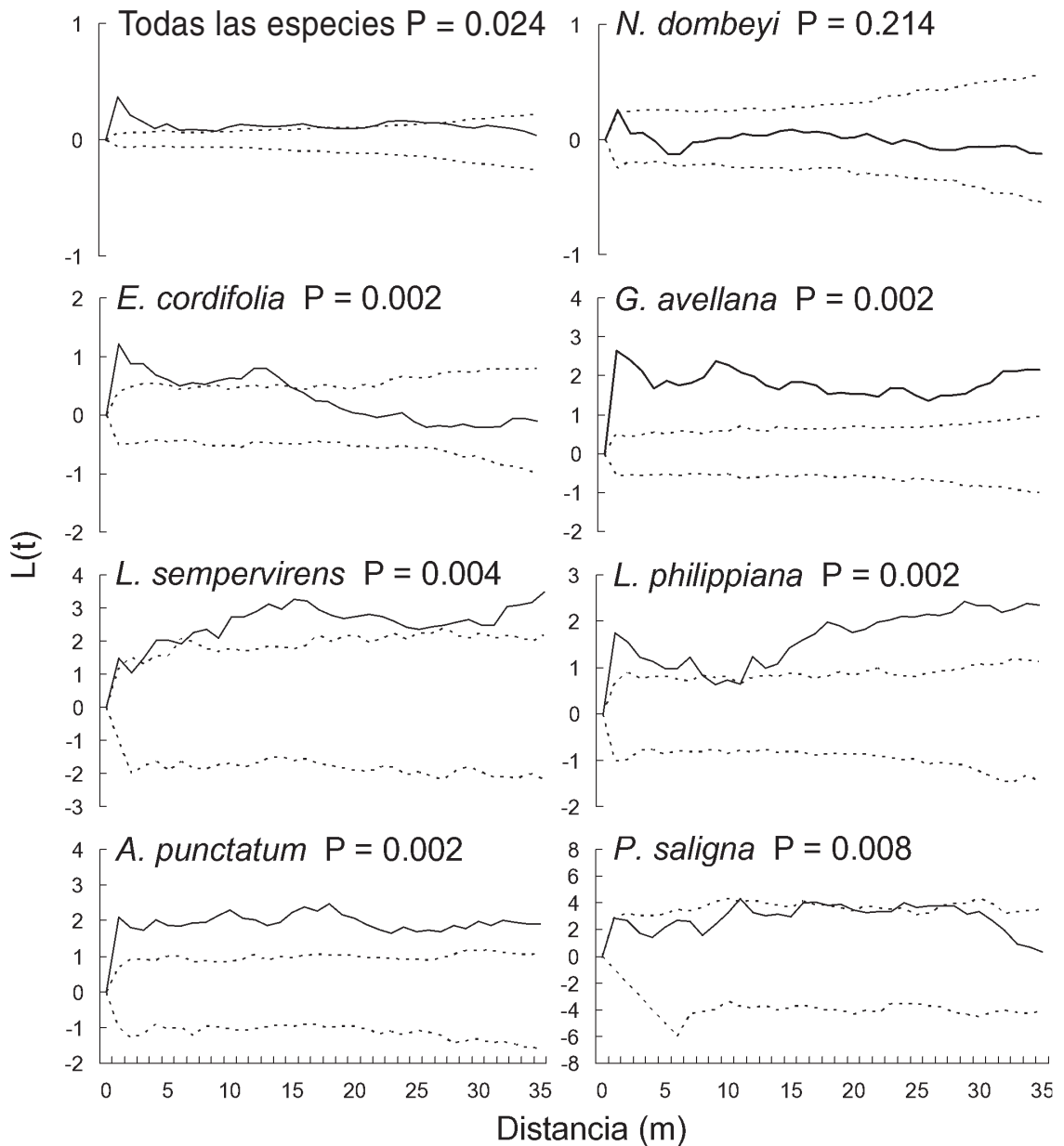
Fig. 3: Patrones espaciales univariados de la función \hat{K}(t) de Ripley para el bosque de Llancahue. La muestra estadística \hat{L}(t) es mostrada por la línea sólida, así como 95 % de intervalos de confianza para el proceso espacial aleatorio está dado por línea punteada.
