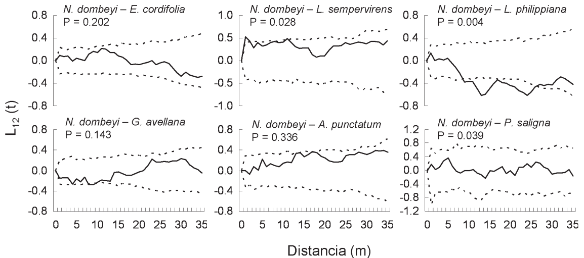
Fig. 4: Asociación espacial biviada de la función \hat{K}_{12}(t) de Ripley para N. dombeyi con las principales especies arbóreas del bosque de Llancahue. La muestra estadística \hat{L}_{12}(t) se muestra con la línea sólida, así como del 95 % de intervalos de confianza para el proceso de indiferencia espacial esta dado por líneas punteada.
