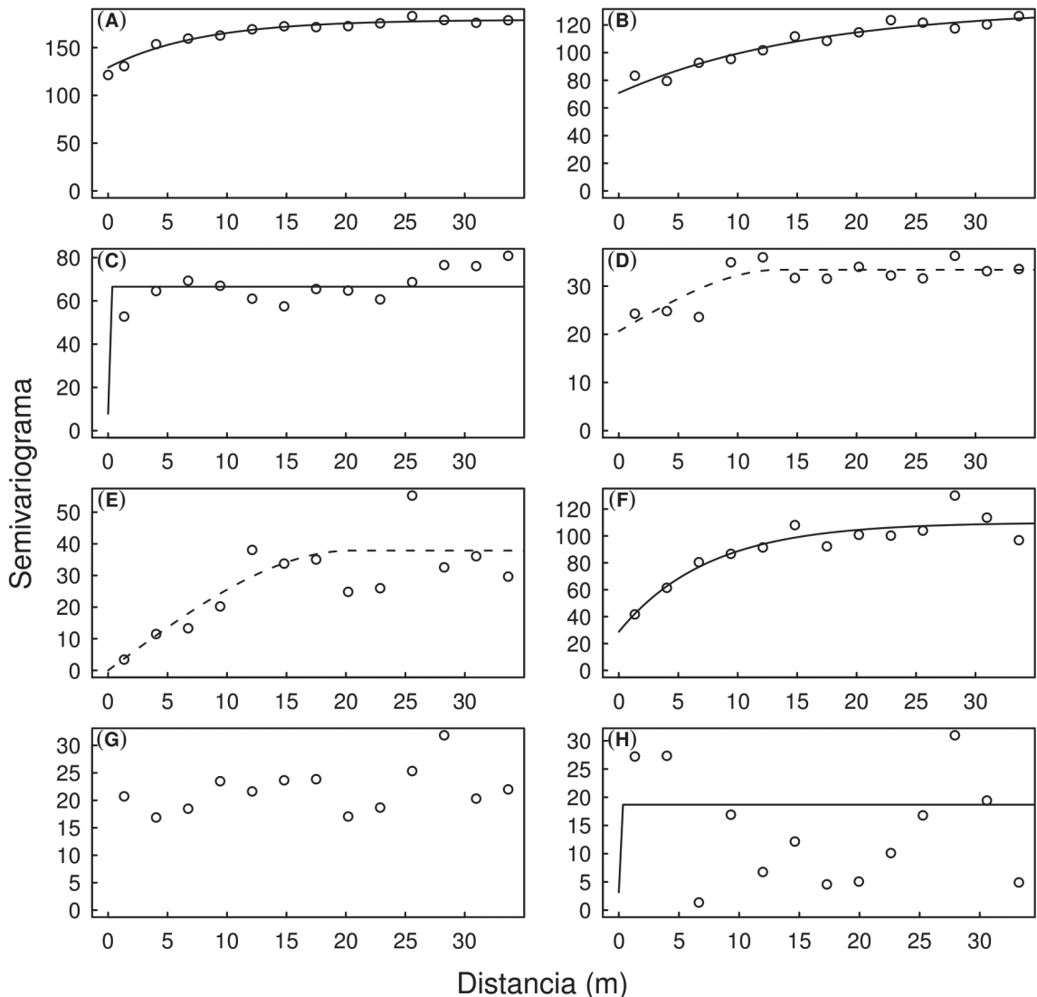
Fig. 5: Semivariogramas empíricos (puntos) y paramétricos (Exponencial: línea sólida; Esférico: línea discontinua; Gaussiana: línea punteada) para el d de los árboles de A) todas las especies, B) N. dombeyi , C) E. cordifolia , D) G. avellana , E) L. Sempervirens , F) L. philippiana , G) A. punctatum , y H) P. saligna .
